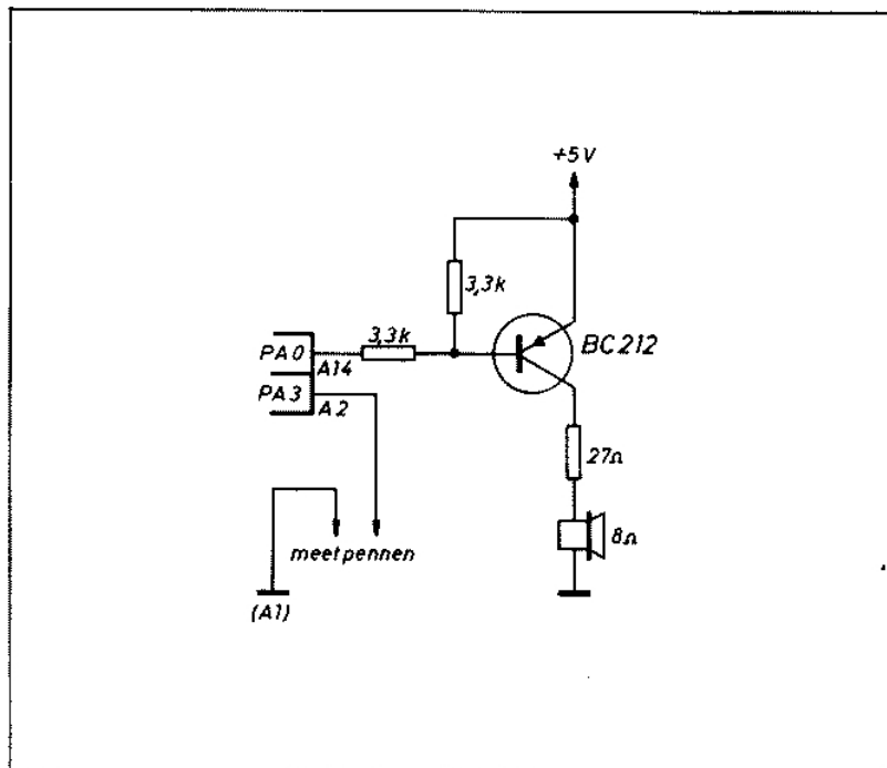
Afb. 1: De aansluitingen welke voor de doormeezoemer gemaakt moeten worden.
