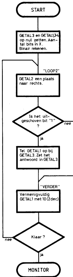
Afb. 1: Het flowdiagram voor de 16-bits vermenigvuldiging.
