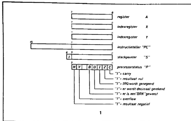
Afb. 1: De inwendige registers van de 6502. Registers Y, PC en S zijn hiervan nog niet besproken.
