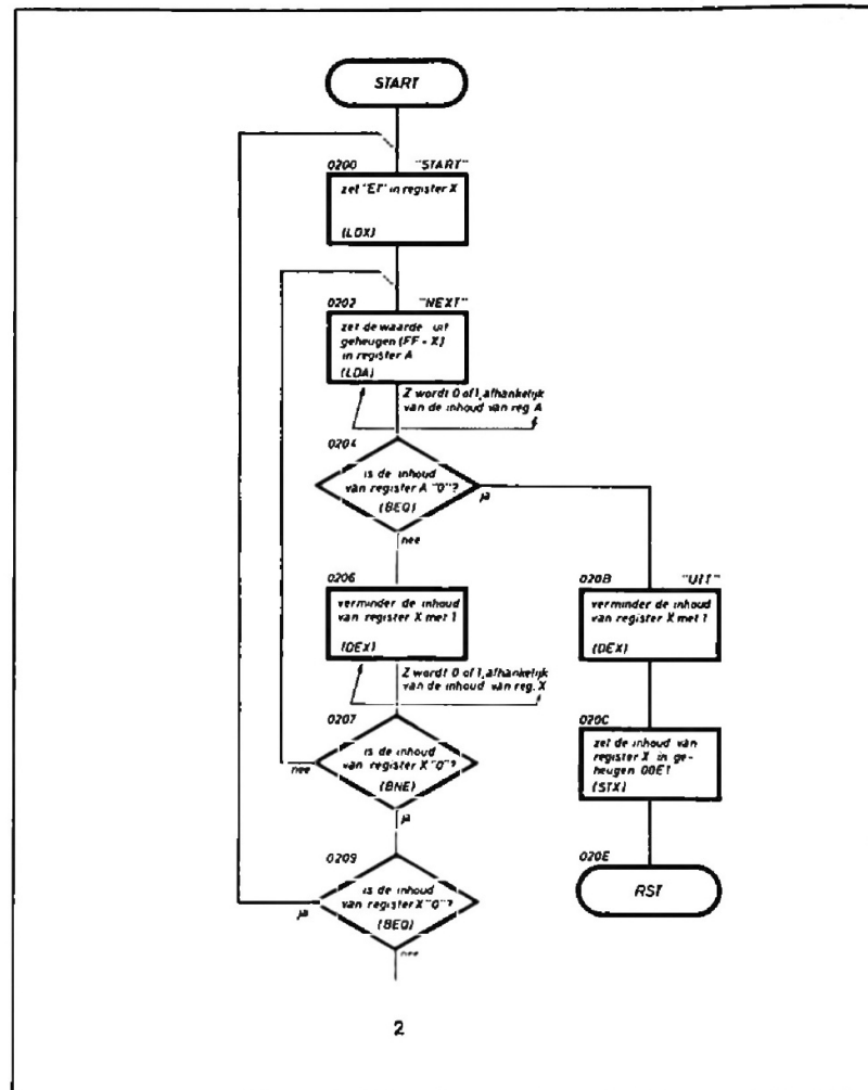
Afb. 2: De flowchart van het op één na laatste voorbeeld. Omdat een flowchart een veel beter overzicht van het programmaverloop geeft, wordt altijd éérst een flowchart gemaakt.
